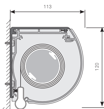
RULLGARDIN (L) MED KASSETT
