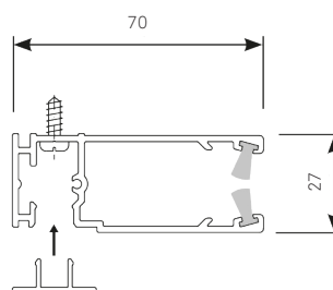
SIDOSLUSS TILL RULLGARDIN (L)
