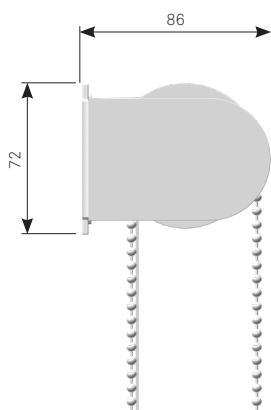
RULLGARDIN (L) STANDARDUTFÖRANDE
