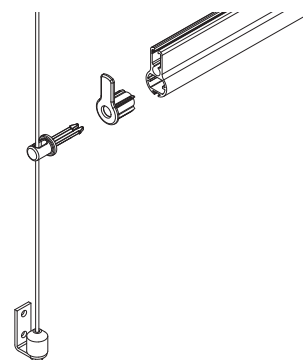
RULLGARDIN (L) MED SIDOSTYRNING WIRE
